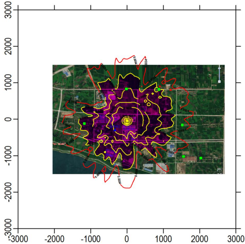
图 6-3 硫化氢小时浓度贡献值分布图
