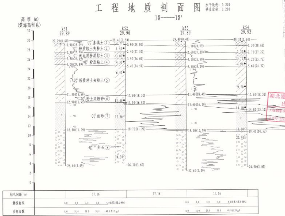
图 6-10 工程地质剖面 1
