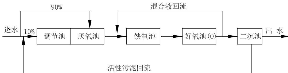
改良 A 2 /O 工艺流程图
