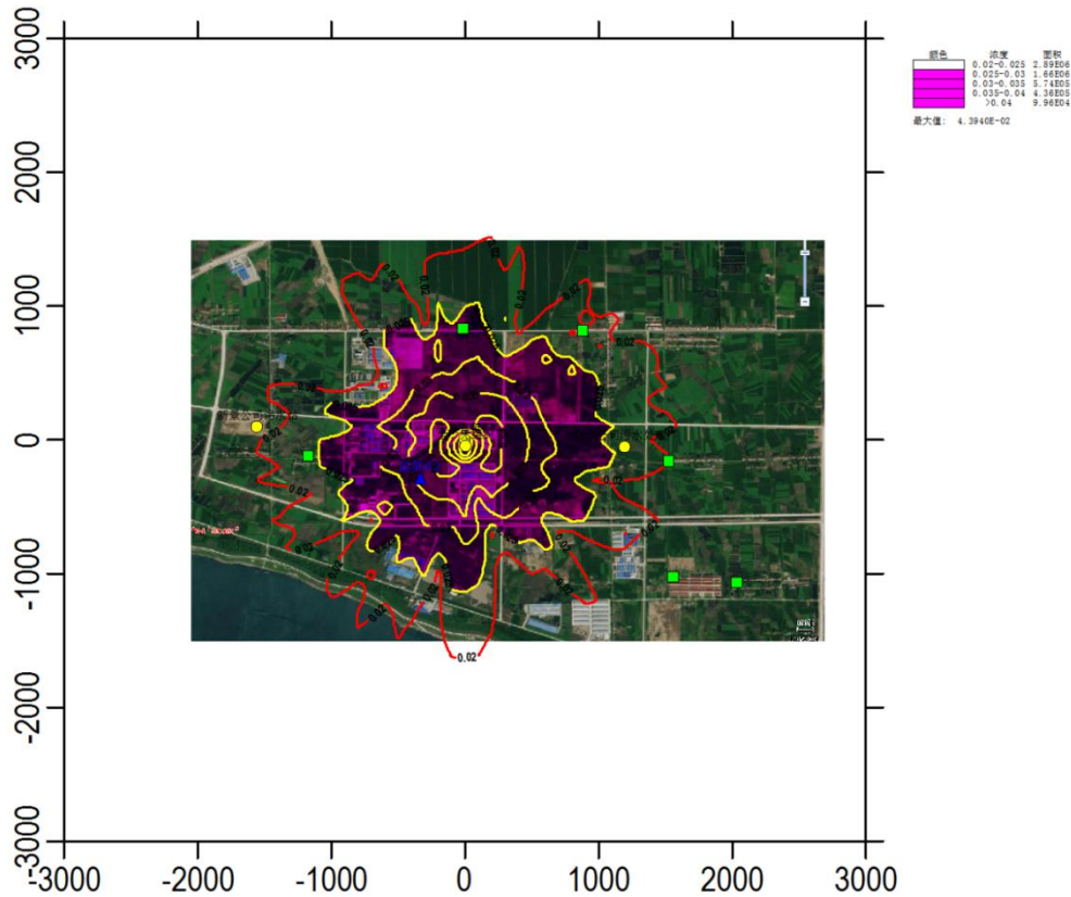
图 6-4 氨小时浓度预测值分布图
