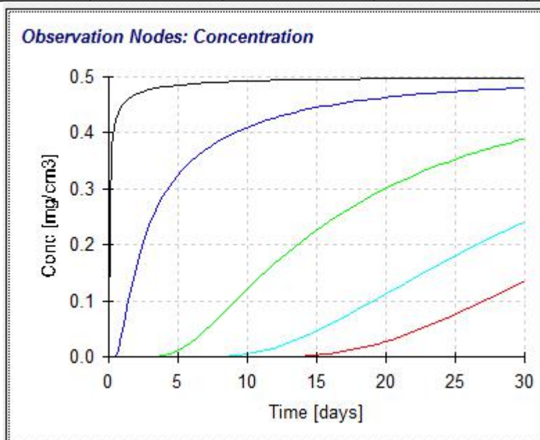
图 6-12不同深度处 COD 污染物浓度随时间变化曲线
