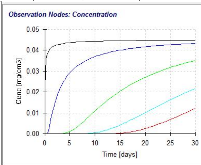
图 6-13 不同深度处氨氮污染物浓度随时间变化曲线
