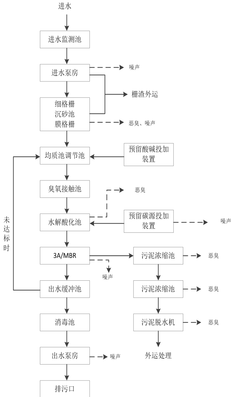
图 2-1 污水处理厂一期工艺流程图
