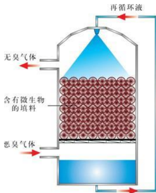
图 8-1生物除臭装置图
