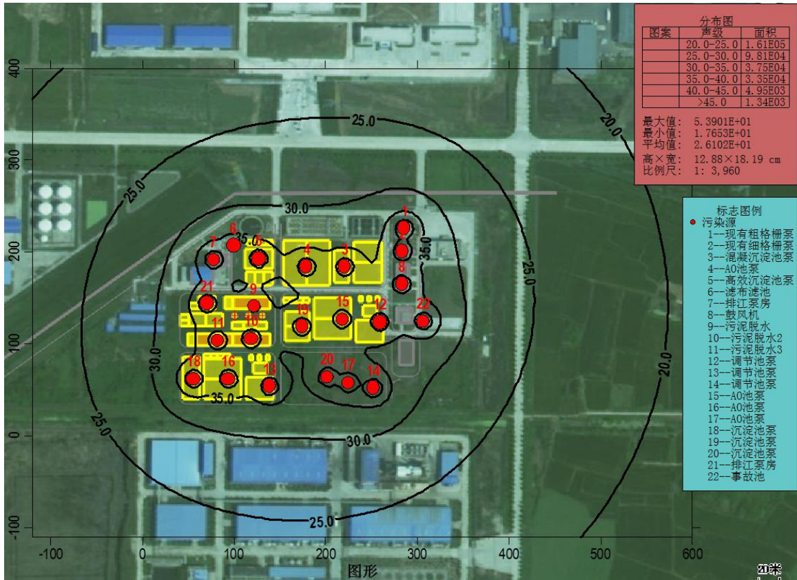
图 6-8 噪声贡献值等值线分布图
