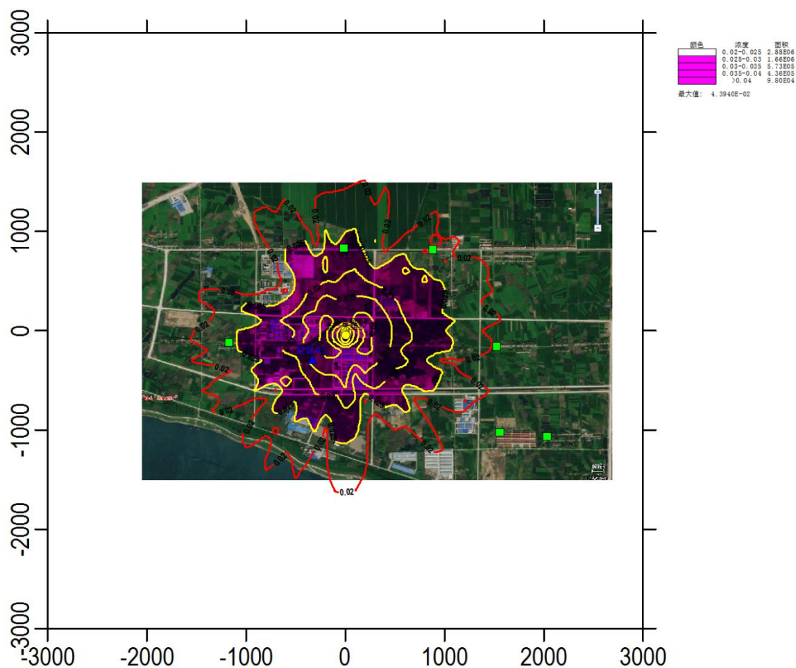
图 6-2 全厂氨小时浓度贡献值分布图
