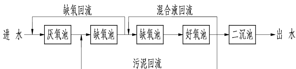
改良型 UCT 工艺流程图
