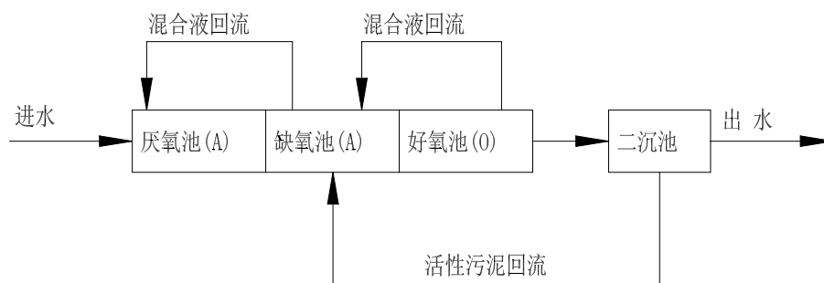
UCT 工艺流程图
